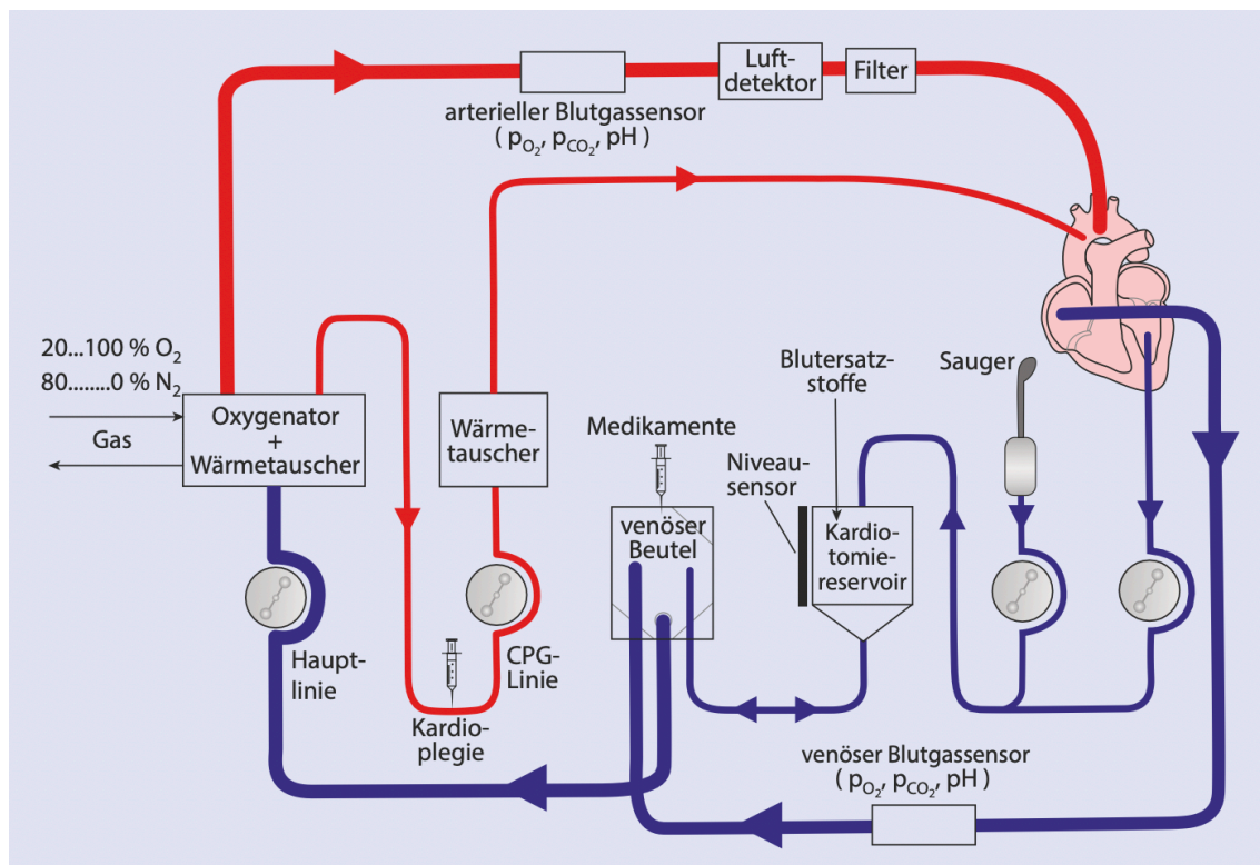
Abb. 8: Schema der extrakorporalen Zirkulation. Das gesamte venöse Blut wird an den Oxygenator der HLM geleitet und von dort in die Aorta oder A. femoralis zurückgepumpt. Die Blutflussrichtung folgt der schematischen Pfeilrichtung. Abb. aus [47].
