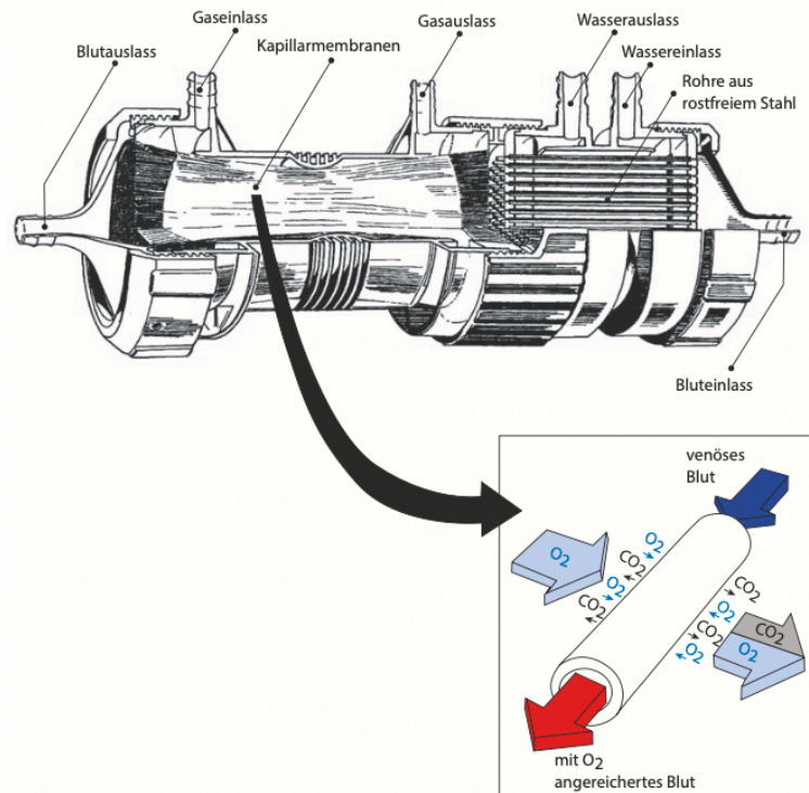
Abb. 9: Kapillarmembranoxygenator. Ein Oxygenator (Bentley) mit integriertem Wärmeaustauscher; schematischer Aufbau. Vergrößerung rechts unten: Die Gase diffundieren durch die Membran in das durch die Kapillaren fließende Blut. Abb. aus [47].
